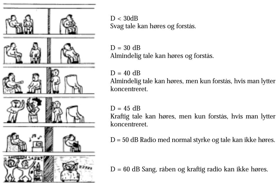
Fig. 6. Sammenhæng mellem rumisolering målt i dB og hørbarheden mellem rum.
