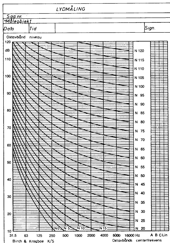
Fig. 11. N-kurver – Noise Rating – er et system af kurver over støjníveauer pr. 1/1 oktav som funktion af frekvensen. Et ønsket støjníveau angives ved en N-værdi, og den tilsvarende kurve angiver den øvre grænse for støjníveauet. I skemaet er angivet nogle N-værdier, som anses for passende i forskellige typer af rum.
