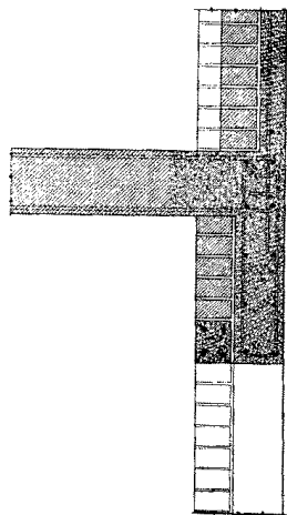
Fig. 6. Færdigstøbt Planke af Jernbeton til Bæring af varmeisolerende 1/2-stens Murværk i Jernbetonhus. Planken armeres i alle fire Hjørner, saa Fejlmontering er udelukket og der ingen Brud kan indtræde under Oplægningen. Plankens Længde er 22 cm større end Vinduesbredden.
