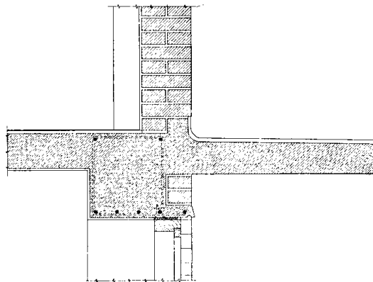
Fig. 10. Vinduesbjælke af Jernbeton med Altan og Dæk af Jernbeton. Den synlige Bæreknastr af Jernbeton støbes med Façadesiden i glat Form. Skalmuringen udføres efter Afformningen.
