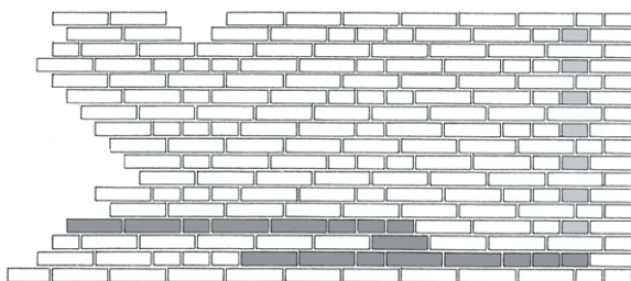
M. forbandt. Kode: 1. sk.: L(0), 2. sk.: 2L+1K+2L+3K(1), 3.sk.: L(-1), 4. sk.: 2L+1K+2L+3K(-1).
