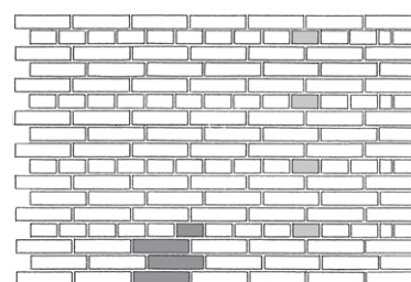
Amerikansk blokforbandt. Kode: 1. sk.: L(0), 2. sk.: L(1), 3.sk.: L(-1), 4. sk.: K(-1).
