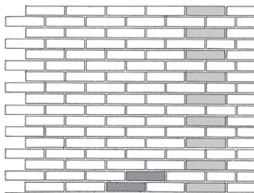
Alm. løberforbandt. Kode: 1. sk.: L(0), 2. sk.: L(2)
