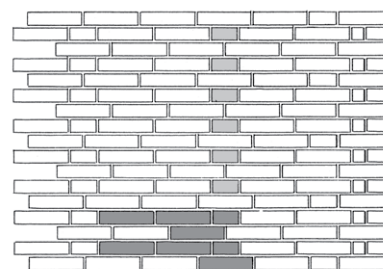
Frederiksbergforbandt. Kode: 1. sk.: L(0), 2. sk.: 2L+1K(1), 3.sk.: L(1), 4. sk.: 2L+1K(-1).
