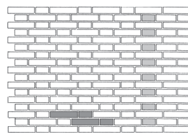
Gotisk munkeforbandt. Kode: 1. sk.: L(0), 2. sk.: L(2).
