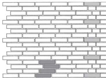
Løberforbandt I. Kode: 1. sk.: L(0), 2. sk.: L(1), 3.sk.: L(1), 4. sk.: L(-1).
