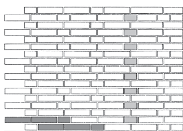
Gl. munkeforbandt. Kode: 1. sk.: 2L+1K(0), 2. sk.: 2L+1K(-5).
