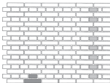
Blokforbandt. Kode: 1. sk.: L(0), 2. sk.: K(-1).
