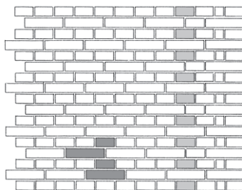
Krydsforbandt. Kode: 1. sk.: L(0), 2. sk.: K(-1), 3.sk.: L(-1), 4. sk.: K(1).
