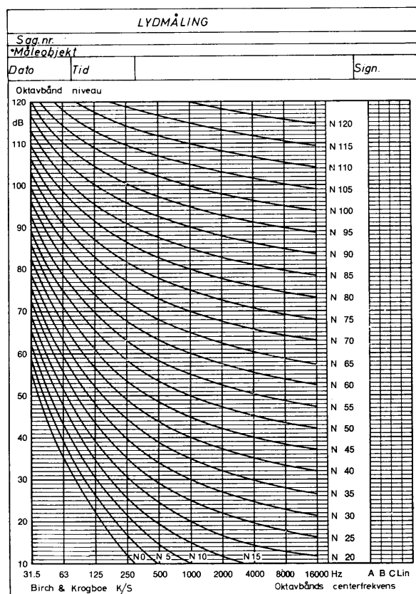
Fig. 11. N-kurver – Noise Rating – er et system af kurver over støjniveauer pr. 1/1 oktav som funktion af frekvensen. Et ønsket støjniveauer angives ved en N-værdi, og den tilsvarende kurve angiver den øvre grænse for støjniveauer. I skemaet er angivet nogle N-værdier, som anses for passende i forskellige typer af rum.
