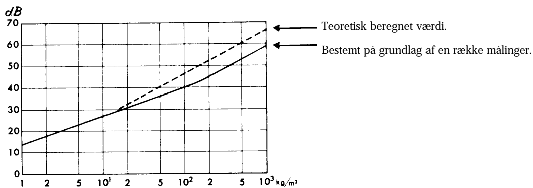
Fig. 8. Reduktionstal som funktion af vægten pr. m 2 .
