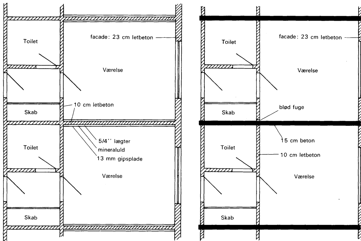
Plan af den første opførte bygning Fig. 9. Lydisolering i et plejehjem.
