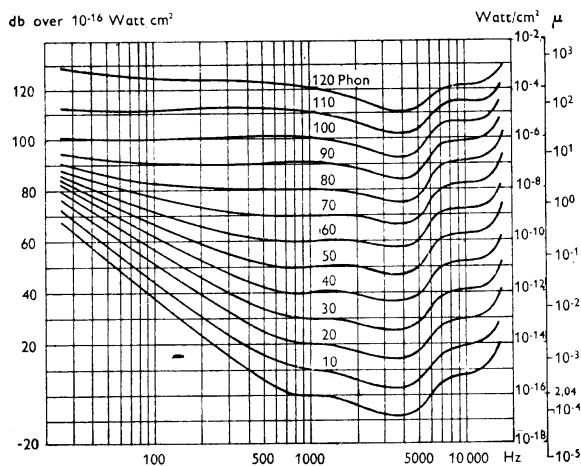
Fig. 3. Fletcher-Munson ørefølsomhedskurver, der angiver ørets følsomhed over for rene toner.
