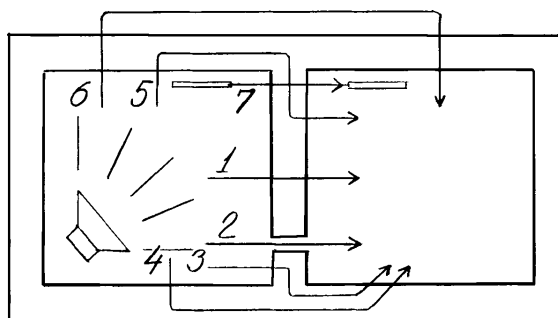
Fig. 5. Forskellige veje for luftlydstransmission mellem to naborum:
