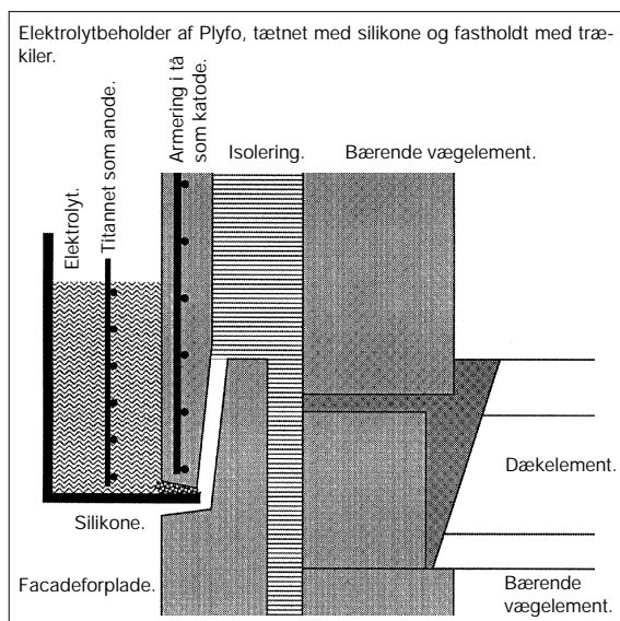
Fig. 6. Eksempel på et arrangement for elektro-kemisk realkalisering af carboniseret »tå« af et facadeelements forplade. Her påsættes en beholder til elektrolyt og anode, men der er også andre muligheder.
