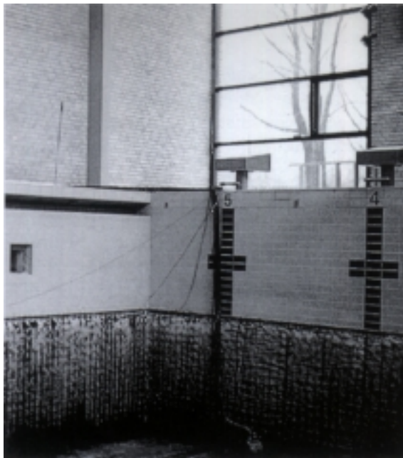
Fig. 7. Hvor det er store betonflader, der skal realkaliseres eller afsaltes (chloridudtrækning), påsprøjtes en gennemvædet cellulosemasse (elektrolyt), hvori anoden placeres, jf. figur 10. Metoden er egnet til chloridudtrækning i svømmebassiner og til realkalivering af facader.
