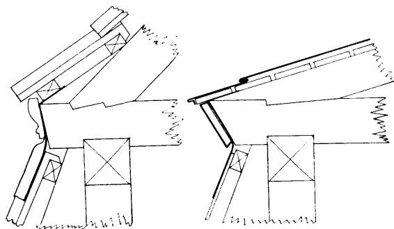
Fig. 9. Sternbaand ved Tegltag og ved Zinktag.
