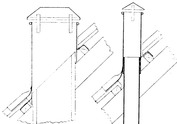
Fig. 20. Inddækning af Lufthætte.
