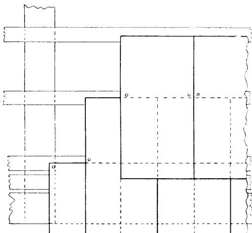
Fig. 14. Retangulær Skiferdækning.
