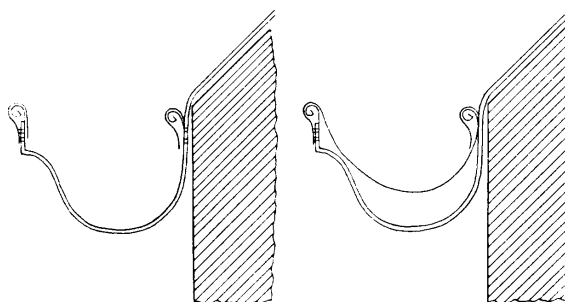
Fig. 3. Karnisrender uden og med Foer.
