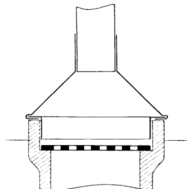
Fig. 8. Skydestykke med Tragt og Rand.
