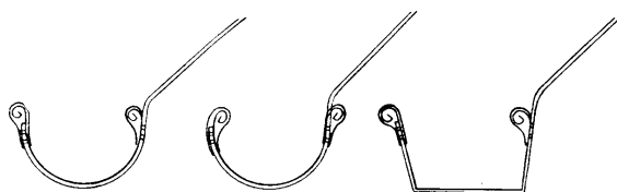
Fig. 1. Halvrunde Render med udføjet og indadløjet vulst.
