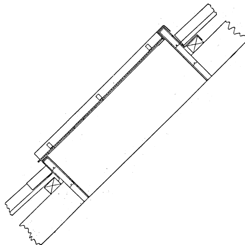
Fig. 18. Ovenlys.
