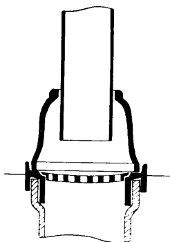
Fig. 6. Klokke og Rand ved Støbejernrør.
