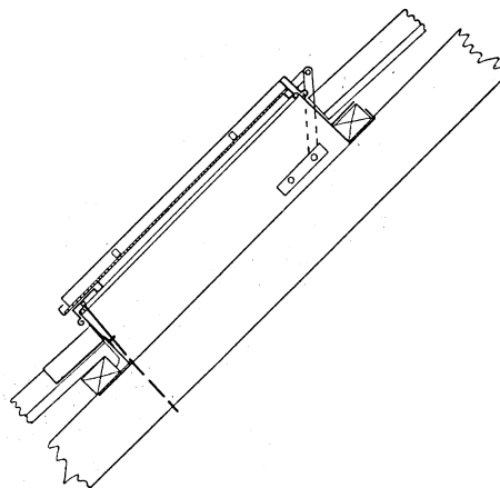
Fig. 19. Tagvindue.
