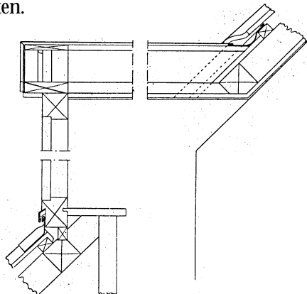
Fig. 17. Kvistedækning.
