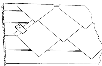
Fig. 15. Stormklammer (ved diagonal Asbestcement-Skifer).
